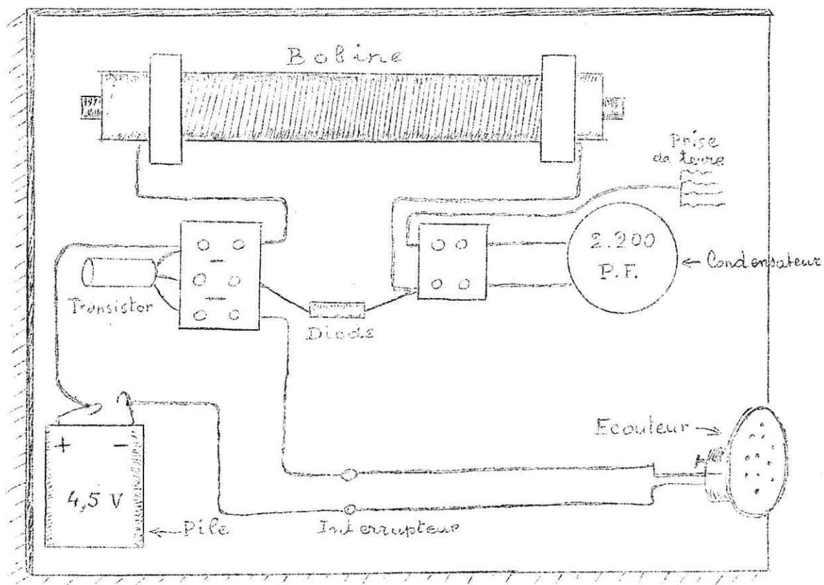
Schema du montage
